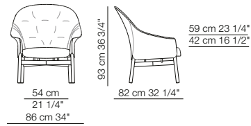
Poltrona con schienale alto trapuntata Quilted armchair with high backrest
