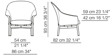
Poltrona con schienale alto Armchair with high backrest
